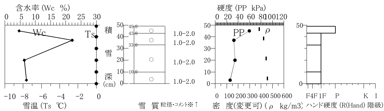
積雪断面観測値 (構内 2019/03/06)
