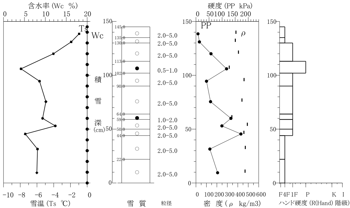
積雪断面観測値 (構内 2021/01/25)
