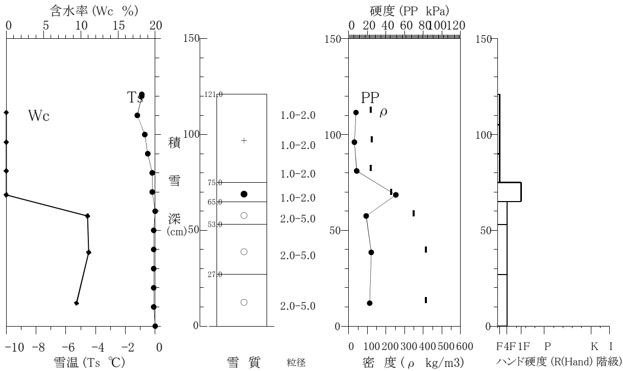
積雪断面観測値 (構内 2022/01/14)
