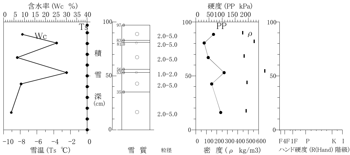
積雪断面観測値 (構内 2022/03/25)
