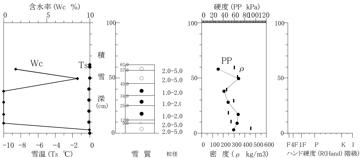
積雪断面観測値 (構内 2023/02/06)
