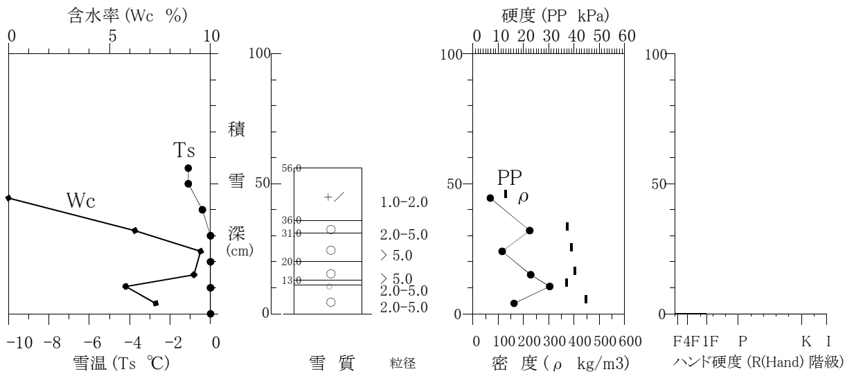
積雪断面観測値 (構内 2023/02/15)
