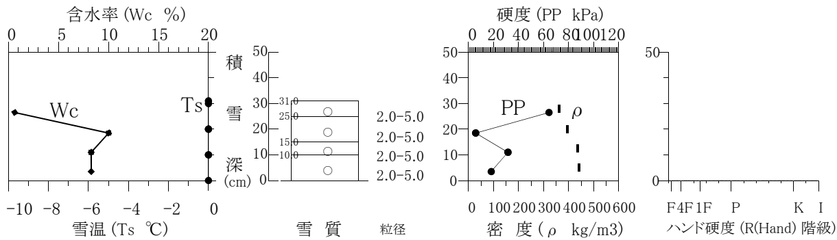
積雪断面観測値 (構内 2024/02/05)
