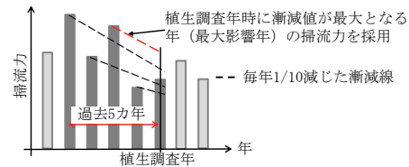
図-2 経過年数を考慮した掃流力の設定
