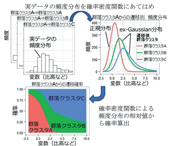
図-3 遷移・更新確率の設定手順
