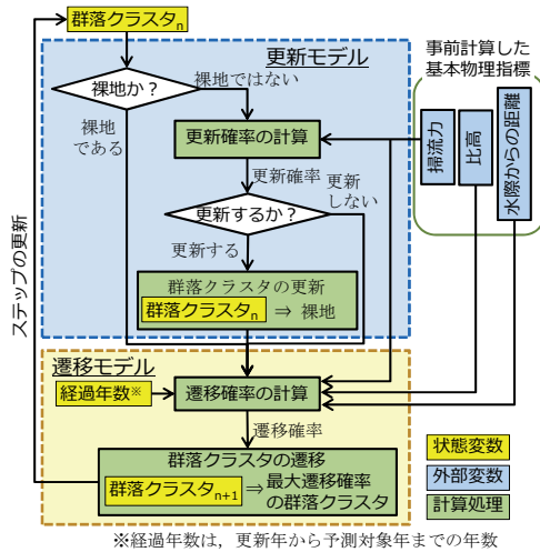
図-5 モデルの計算フロー
